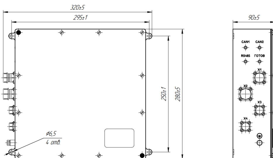
Рис. 4. Фрагмент габаритного чертежа блока сопряжения средств
