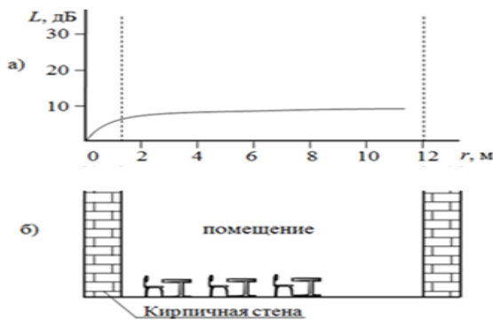
Рис. 3. а) усредненная зависимость ослабления сигнала на частоте 1800 МГц от расстояния в пустом помещении; б) место экспериментального исследования
