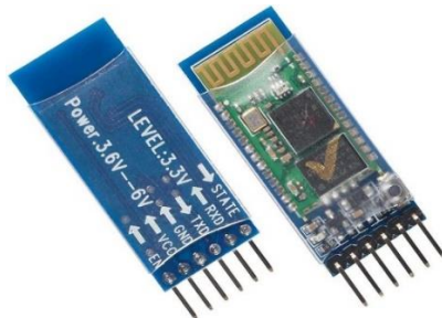
Рис. 3. Bluetooth-модуль HC-05
