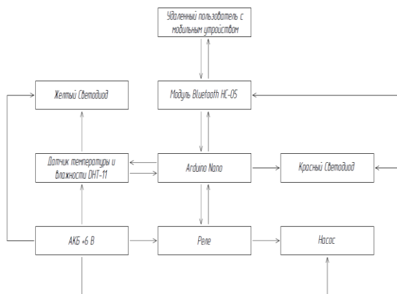
Рис. 5. Структурная схема устройства
