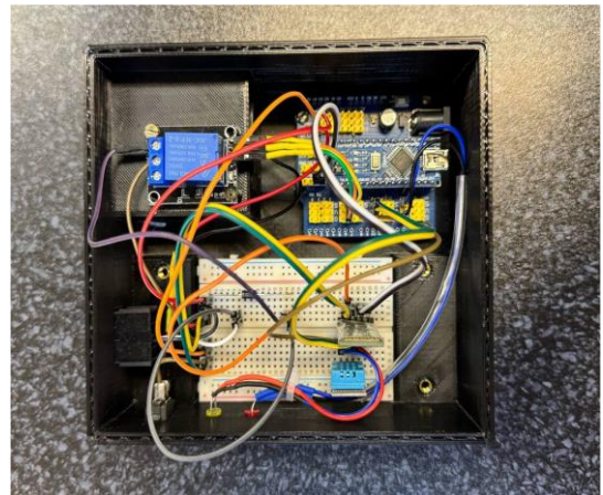
Рис. 8. Фотография опытного образца вид сверху
