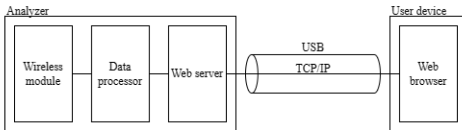
Рис. 1. Высокоуровневая архитектура анализатора
