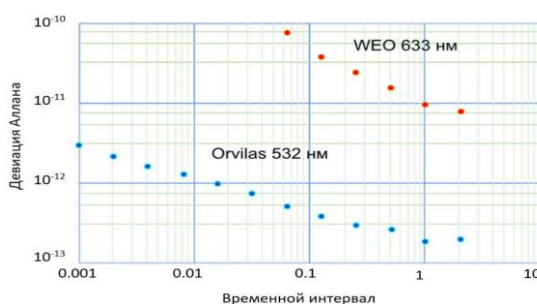
Рис. 3. Кратковременная стабильность частоты малогабаритного лазера Nd:YVO 4 /KTP/I 2 на 532 нм и He-Ne/I 2 лазера на 633 нм
