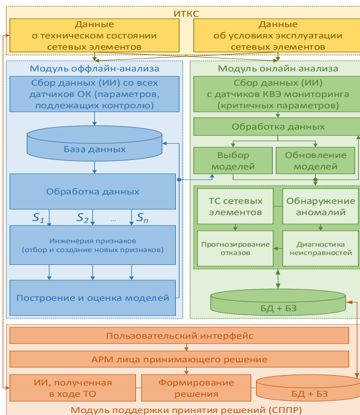
Рис. 2. Предложенная структура процесса сетевого мониторинга
