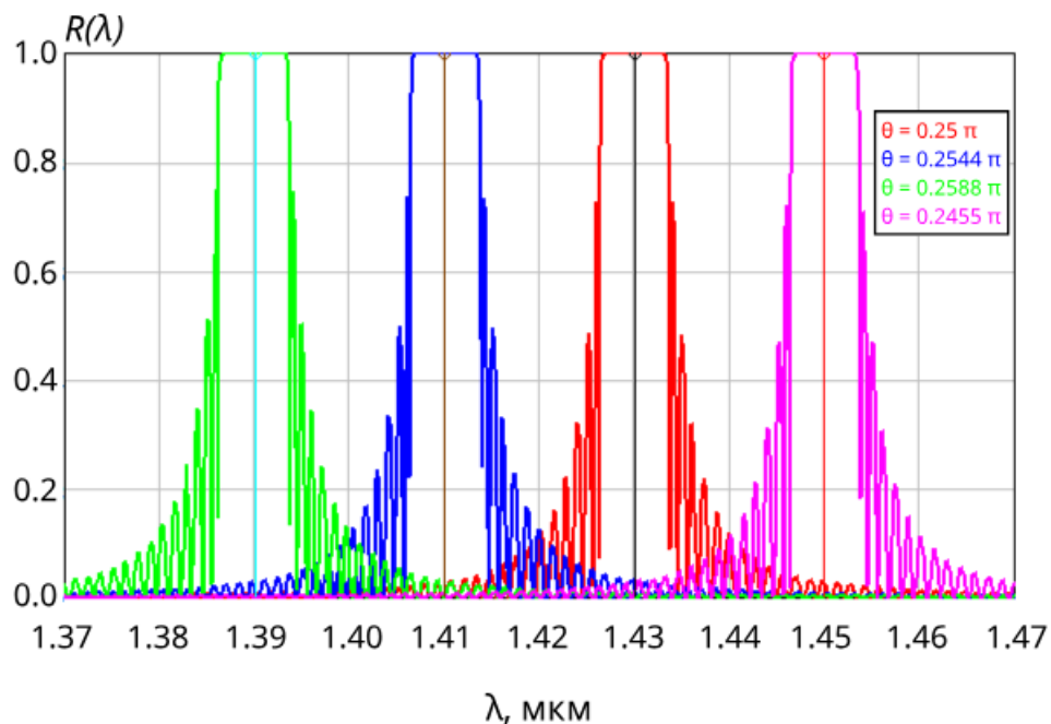
Рис. 5. Спектр отражения от фильтра при разных углах падения светового пучка
