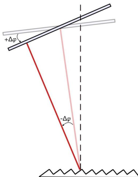
Рис. 2. Поворот зеркала при перестройке длины волны
