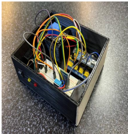
Рис. 7. Фотография опытного образца изометрическая проекция
