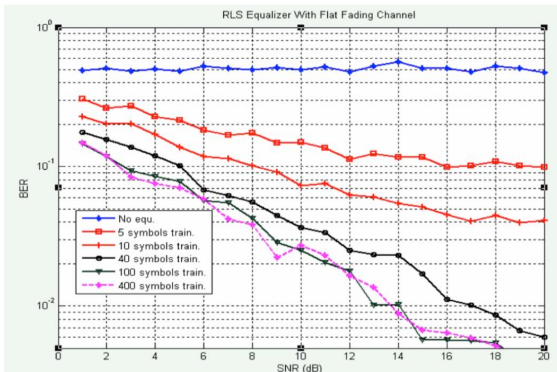
Рис. 3. Зависимость количества битовых ошибок от длины преамбулы [9]
