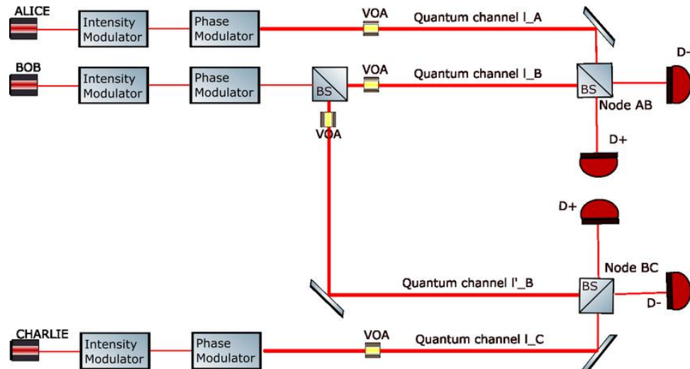
Рис. 1. Протокол TF-QKD
