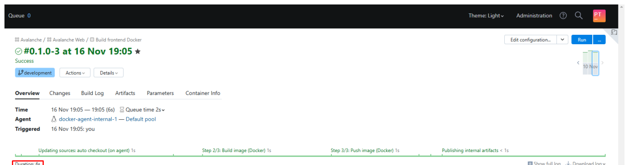
Рис. 3. Сборка пайплайн
