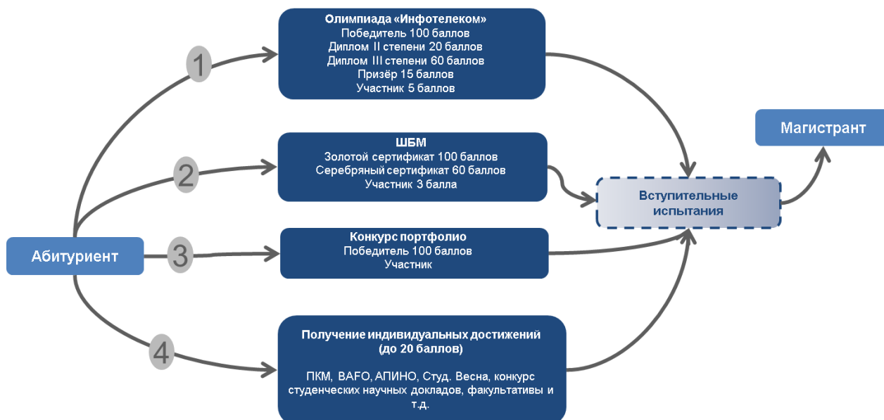
Рис. 1. Траектории поступления в магистратуру
