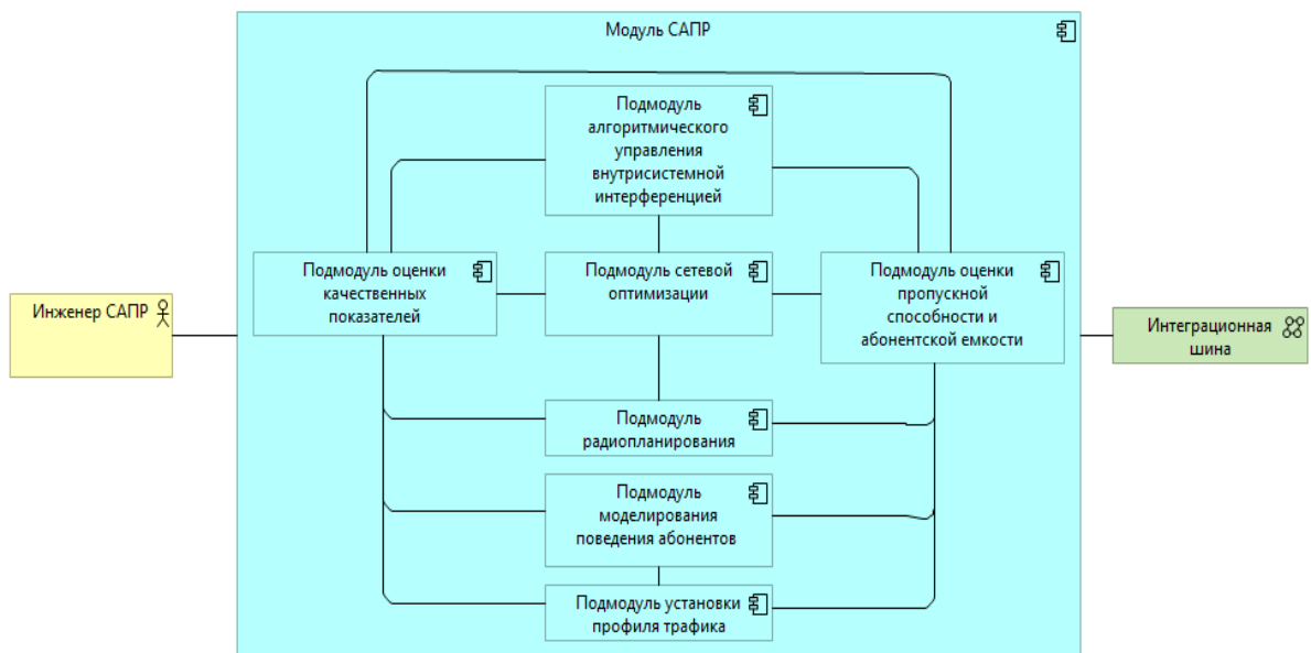
Рис. 2. Структура модуля САПР
