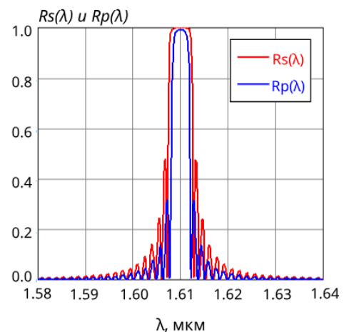
Рис. 4. Спектр отражения от фильтра при разной поляризации света
