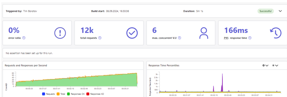
Рис. 2. Результат тестирования системы WFM с помощью инструмента «Gatling»
