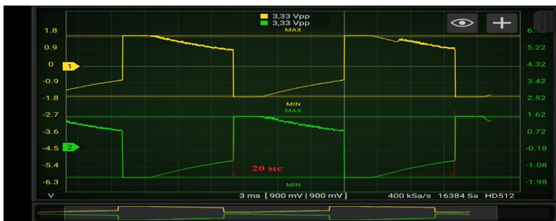
Рис. 5. Осциллограммы сигналов управления 50 Гц транзисторами VT1 и VT2 мостовой резонансной схемы последовательного инвертора
