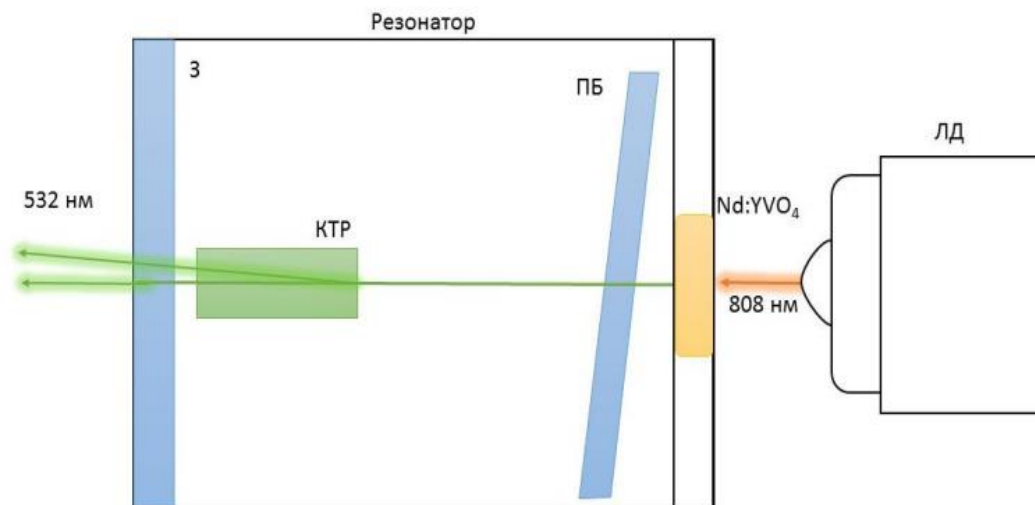
Рис. 2. Оптическая схема лазерного резонатора Nd:YVO 4 /KTP с выходным излучением 532 нм
