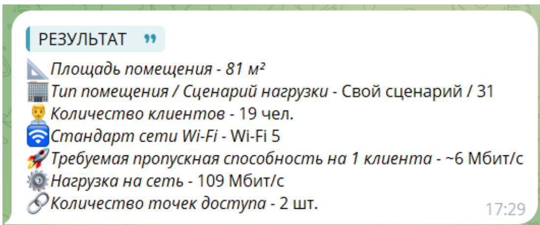
Рис. 3. Результат работы чат-бота
