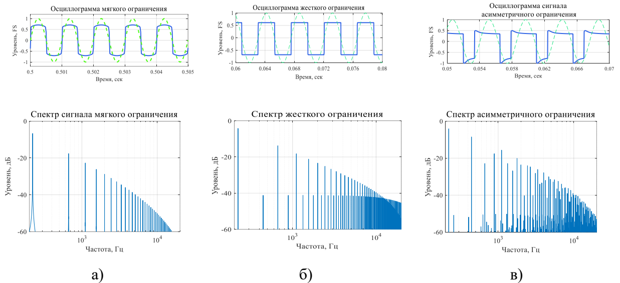
Рис. 4. Схемы, осциллограммы и спектры а) мягкого, б) жесткого, в) асимметричного ограничений
