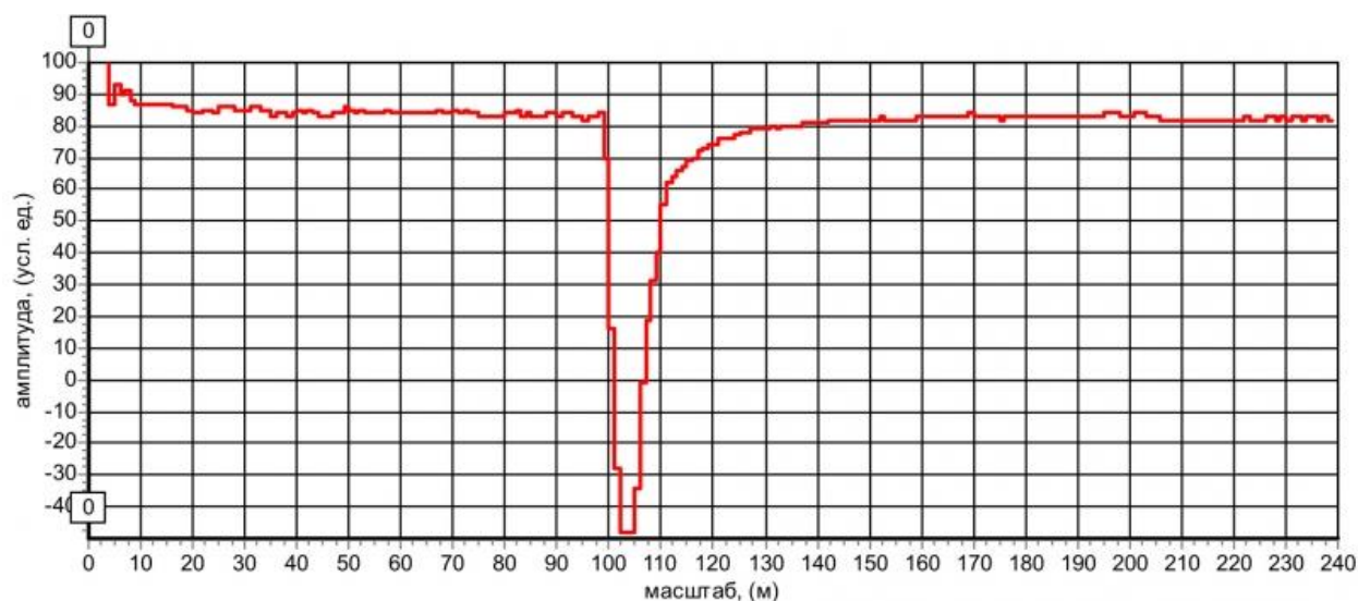
Рис. 3. Рефлектограмма КЛ с неоднородностью типа «полное короткое замыкание»
