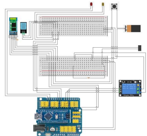
Рис. 6. Принципиальная схема устройства
