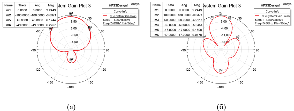
Рис. 4.1. Диаграмма направленности антенной решетки в Е (а) и Н (б) плоскостях
