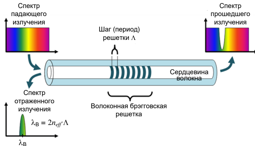
Рис. 1. Однородная ВБР
