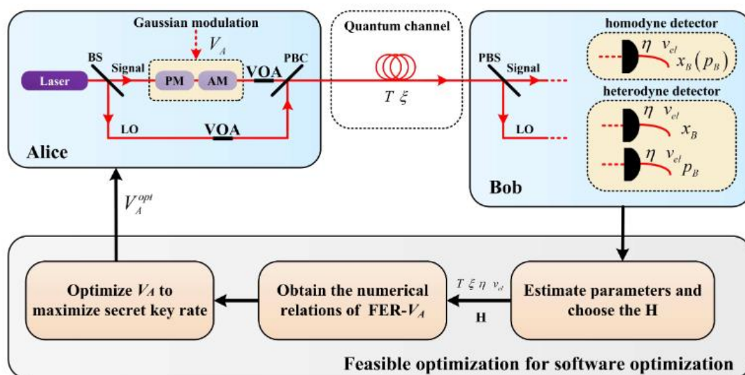
Рис. 2. Протокол CV-QKD
