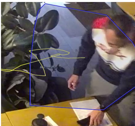
Рис. 1. Обнаружение движения
