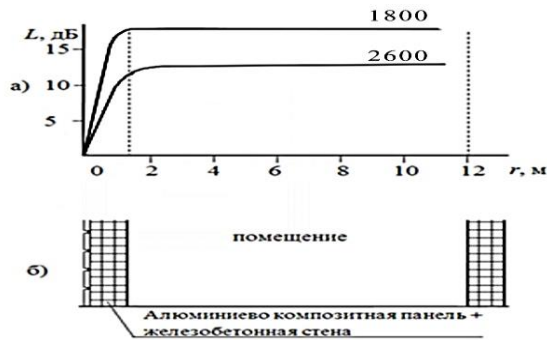
Рис. 1. а) усредненная зависимость ослабления сигнала на частоте 1800 и 2600 МГц от расстояния в пустом помещении; б) место экспериментального исследования
